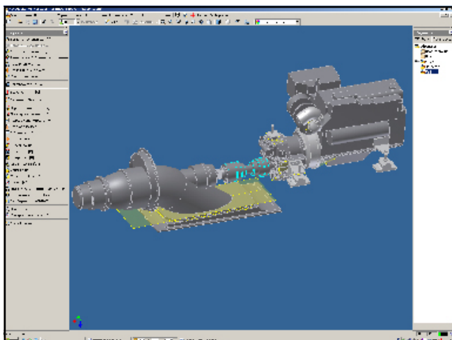
Рис. 5. Стыковка главного двигателя с водометом
