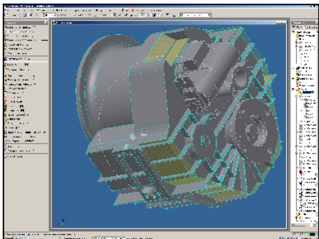
Рис. 7. Редуктор главного двигателя ZF-63
